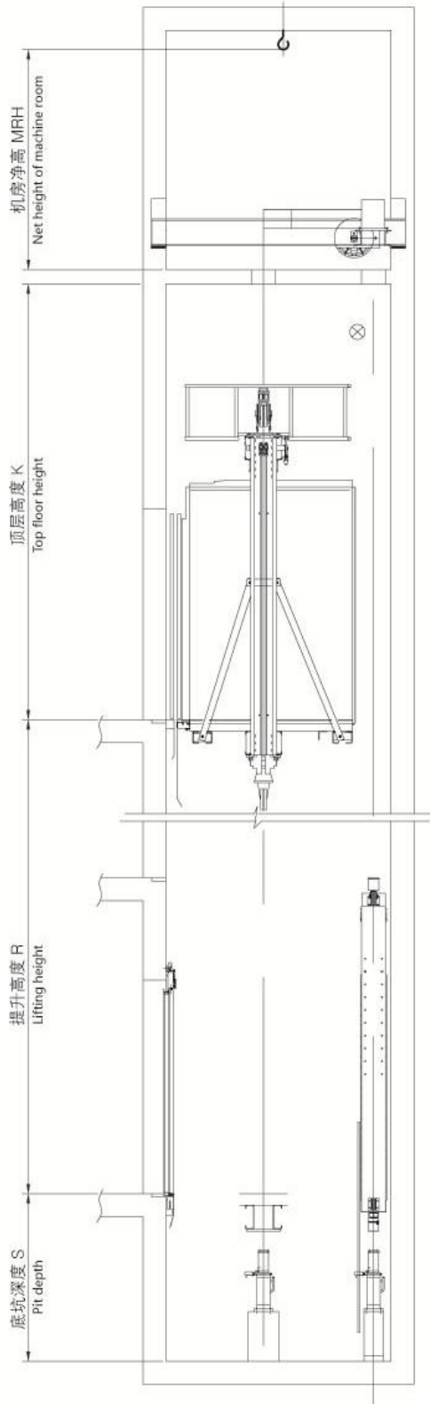
井道立面图 Shaft section plan
