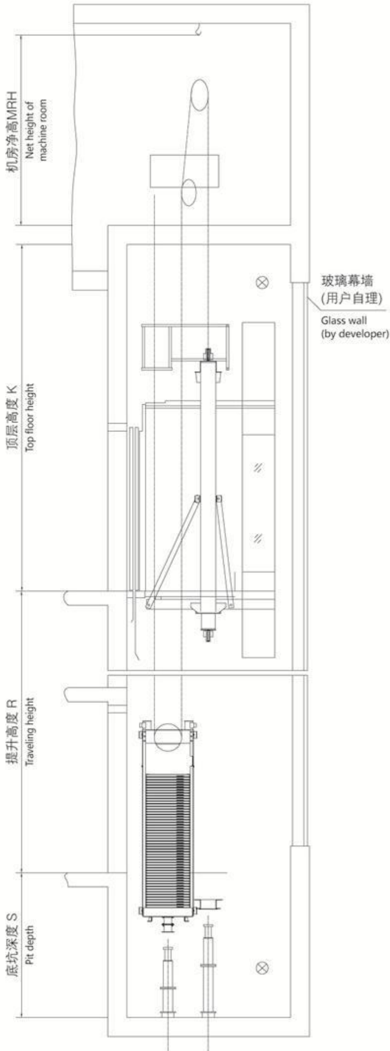
井道立面图 Shaft section plan
